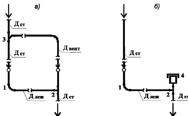
а) с устройством вентиляционного трубопровода (байпаса); б) с установкой автоматического противовакуумного клапана 1 — первая точка изменения направления; 2 — вторая точка изменения направления; 3 — точка подключения вентиляционного трубопровода (байпаса); 4 — автоматический противовакуумный клапан
