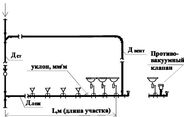
Рисунок 11.2 — Схема устройства длинной горизонтальной разводки
