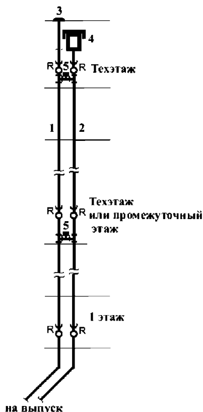
1 — основной водосточный стояк; 2 — резервный водосточный стояк; 3 — водосточная воронка; 4 — автоматический противовакуумный клапан; 5 — перемычка; R — ревизия
